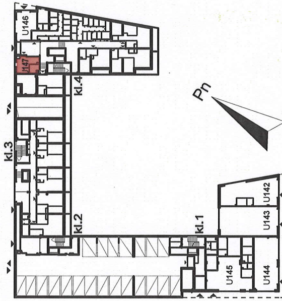
RZUT POZIOMY KONDYGNACJI PIERWSZEJ
